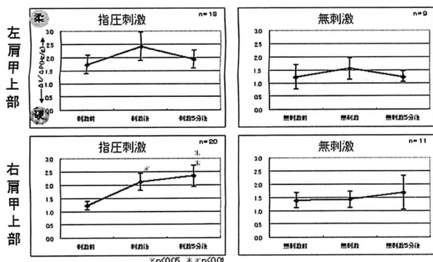
図7 押し込み量対周波数変化
