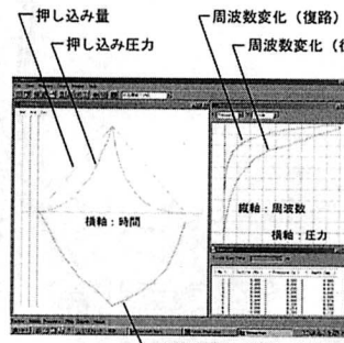
図5 測定画面とエラー判断
